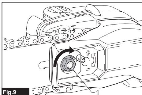
Fig. 9 ► 1. Écrou de retenue
