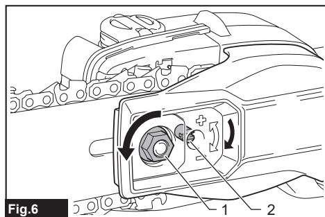
Fig. 6 ► 1. Écrou de retenue 2. Vis de réglage de la chaîne
