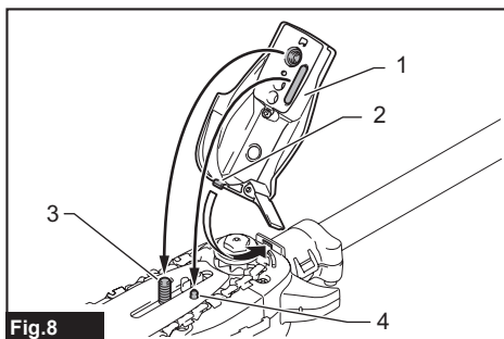
Fig. 8 ► 1. Protecteur de pignon 2. Partie saillante 3. Boulon 4. Broche
