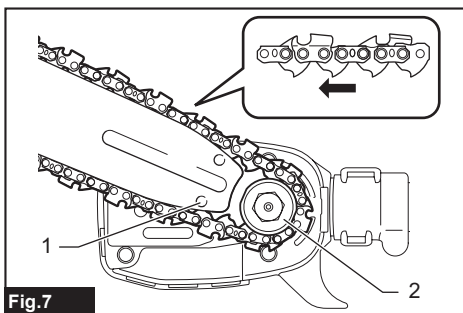
► 1. Hole 2. Sprocket
