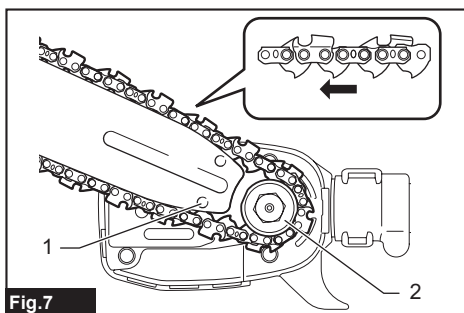
Fig. 7 ► 1. Orifice 2. Pignon
